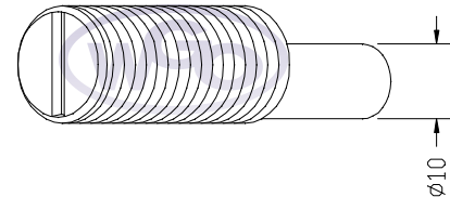
PINO ROSCADO EXCÊNTRICO \varnothing 10mm P/ TB-42 E TB-60
