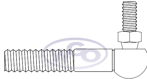
ARTICULAÇÃO ANGULAR P/ CILINDRADOR P/ A-15 E A-25
